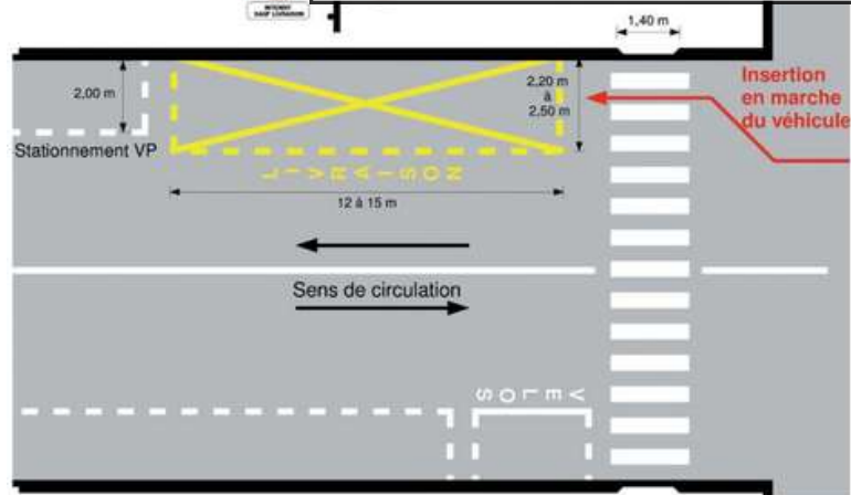
Schéma de principe d'une aire de livraison - Source : CERTU 2013 "Aires de livraison : planifier, aménager et gérer l'accueil des véhicules" - Thomas Plantier
