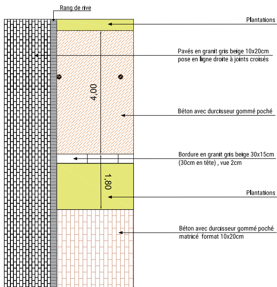
Détail d'agencement sur placette pavée (Détail 1)
